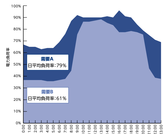
図-1 本学の電力需要場所における負荷率の推移
